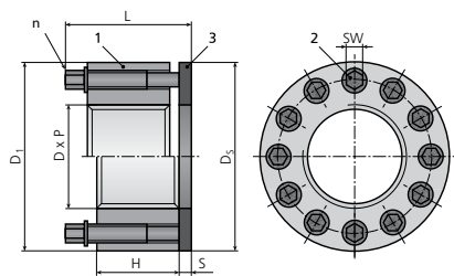
组件: 1. 螺母主体 2. 顶推螺钉 3. 硬化垫圈
